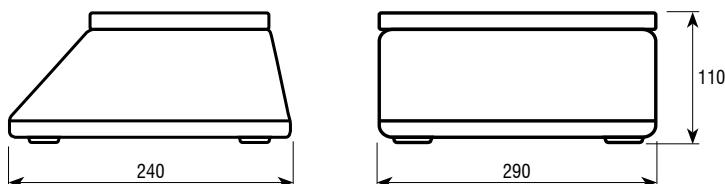
Dimensiones (mm)
